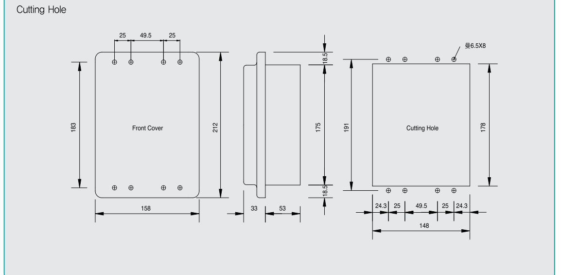
외형치수도
