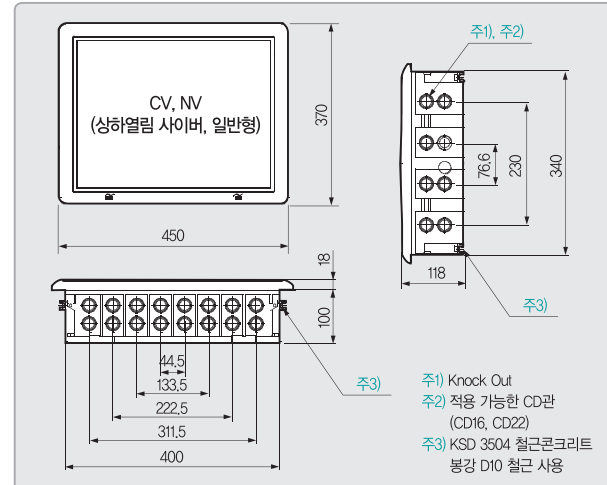
NV516 / NV616 / NV1016
