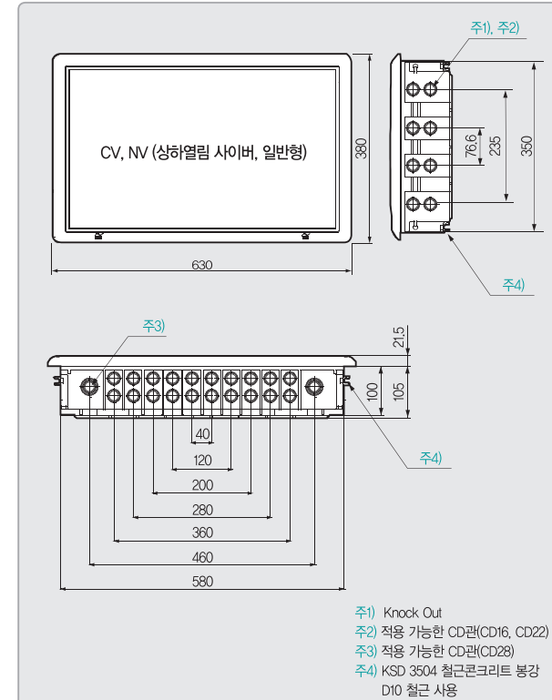
NV526 / NV626 / NV1026
