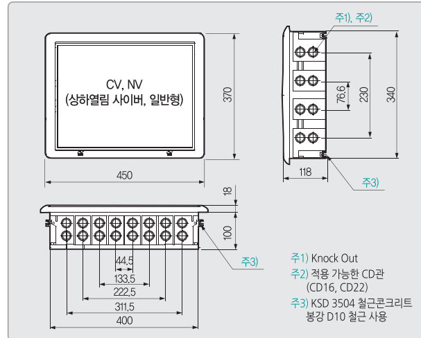
NV522 / NV622 / NV1022
