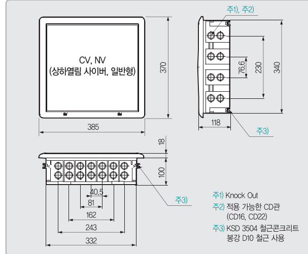
NV516 / NV616 / NV1016
